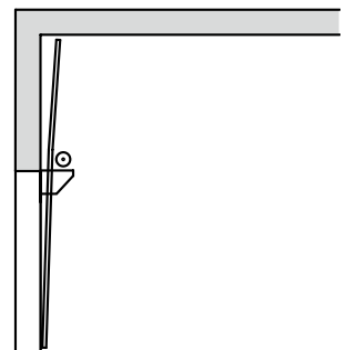
Beschlagsart VU mit unten liegender Federwelle
